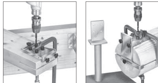
for/pro/pentru: joist and support bracket 90 / skrytá trémová botka 90 / suport grinda 90
